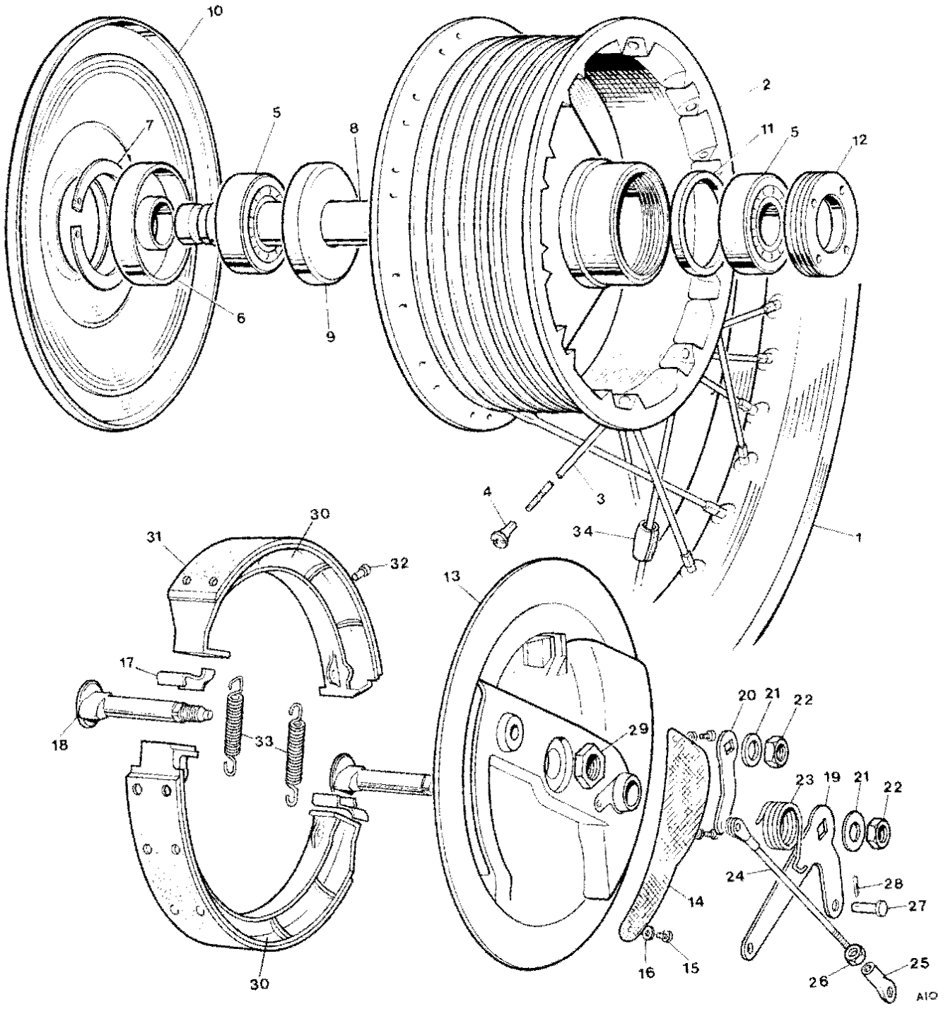
Fig. 10. FRONTWHEEL
