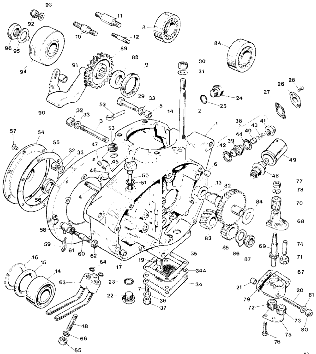
Fig. 2. CRANKCASE
