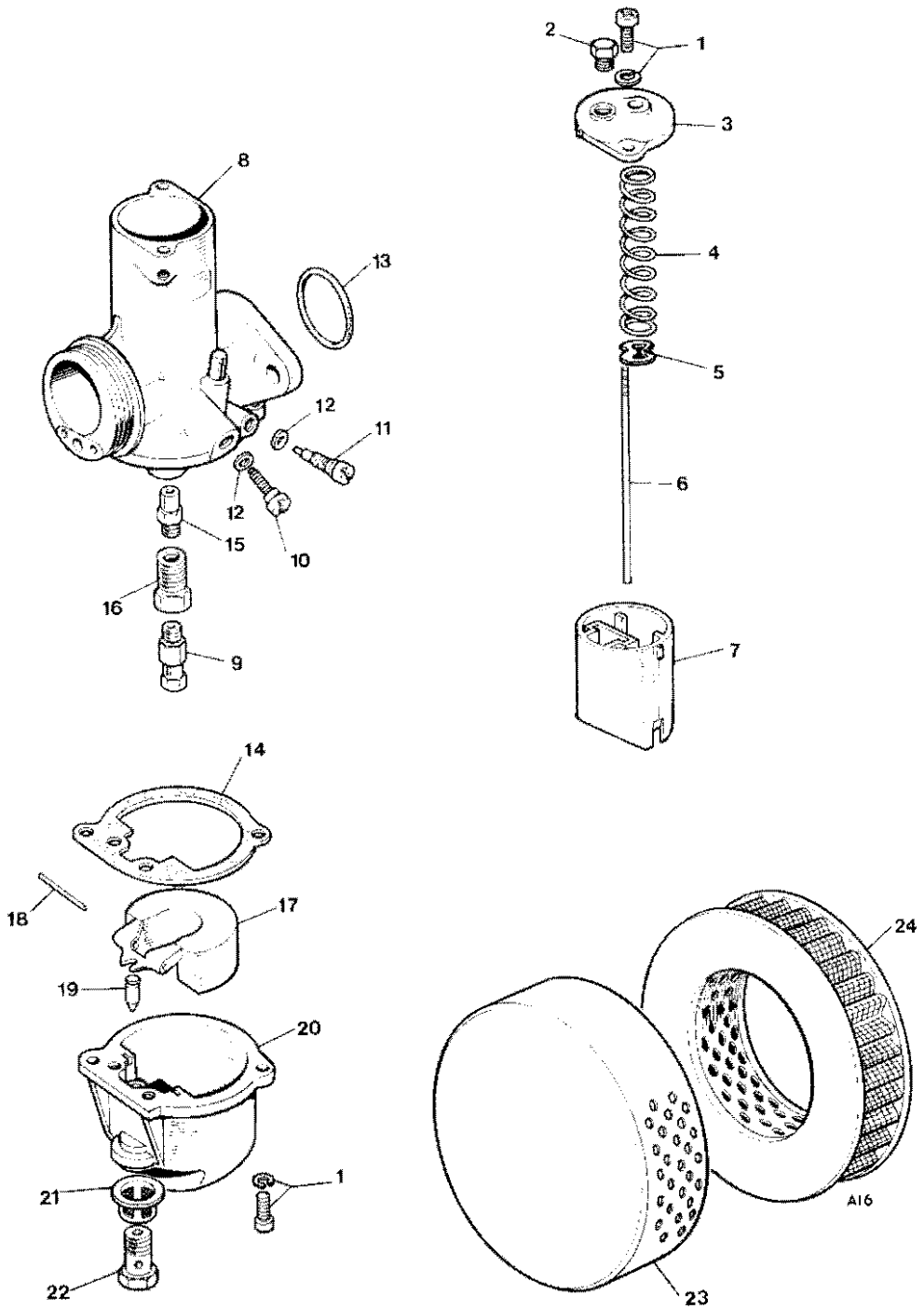
Fig. 18. CARBURETOR
