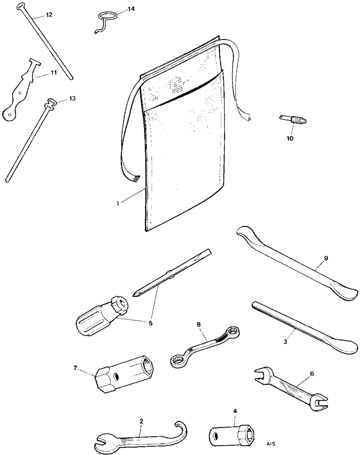
Fig. 17. TOOL KIT
