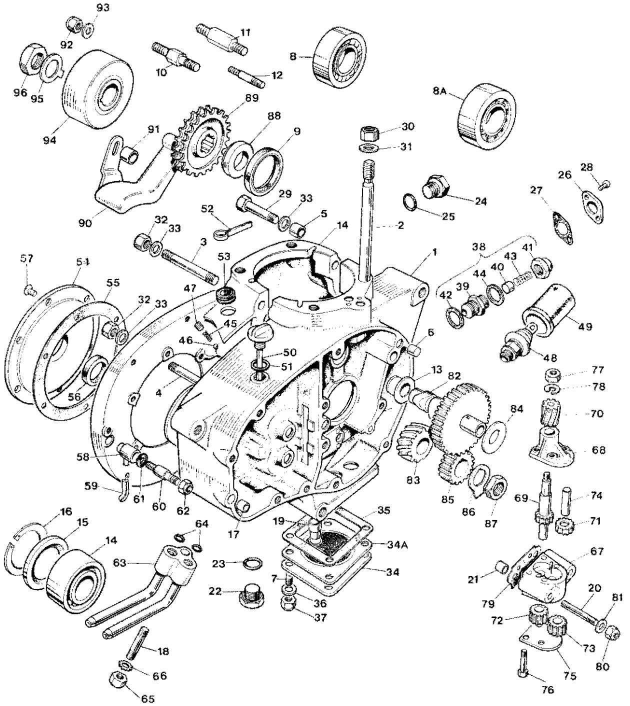
Fig. 2. CRANKCASE
