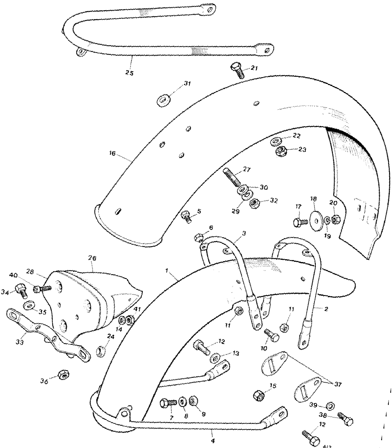
Fig. 12. FENDERS
